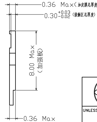
APPLICABLE FPC RECOMMENDED DIMENSION 一体式铝箔加强板排线（接地）
