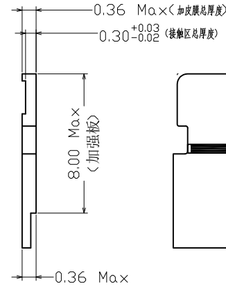
APPLICABLE FPC RECOMMENDED DIMENSION 蓝白裸线（不接地）
