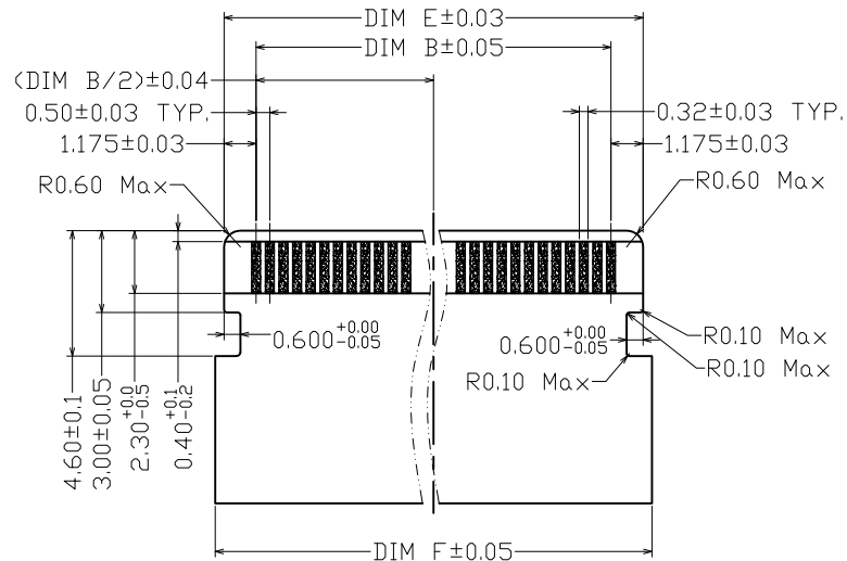
APPLICABLE FPC RECOMMENDED DIMENSION 蓝白裸线（不接地）
