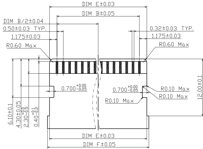
APPLICABLE FPC RECOMMENDED DIMENSION 蓝白裸线（不接地）
