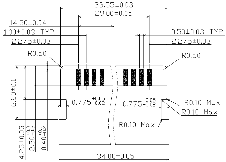
APPLICABLE FPC RECOMMENDED DIMENSION 蓝白裸线（不接地）
