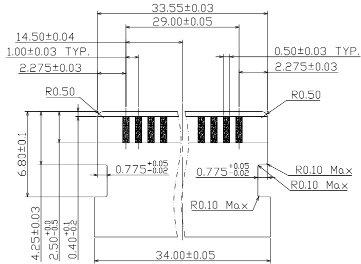
APPLICABLE FPC RECOMMENDED DIMENSION 一体式铝箔加强板排线（接地）
