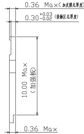
APPLICABLE FPC RECOMMENDED DIMENSION 蓝白裸线（不接地）
